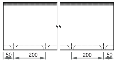
rozkład otworów montażowych w profilu o długości 1500 mm
