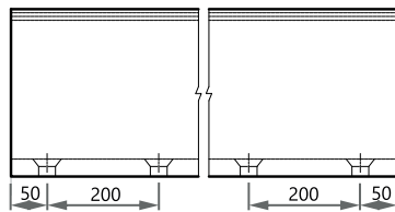
rozkład otworów montażowych w profilu o długości 1500 mm
