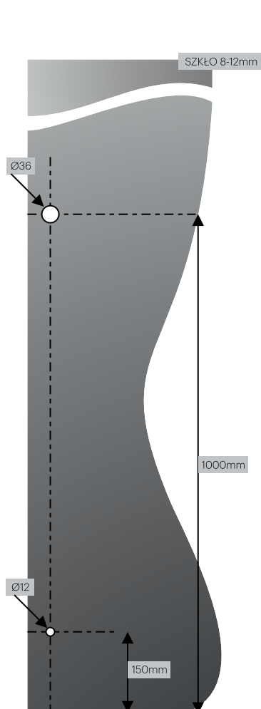
WP30160 wkładka 160/30
