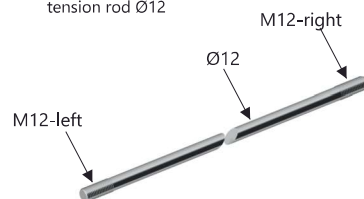
NGDS 6013 tension rod Ø12
